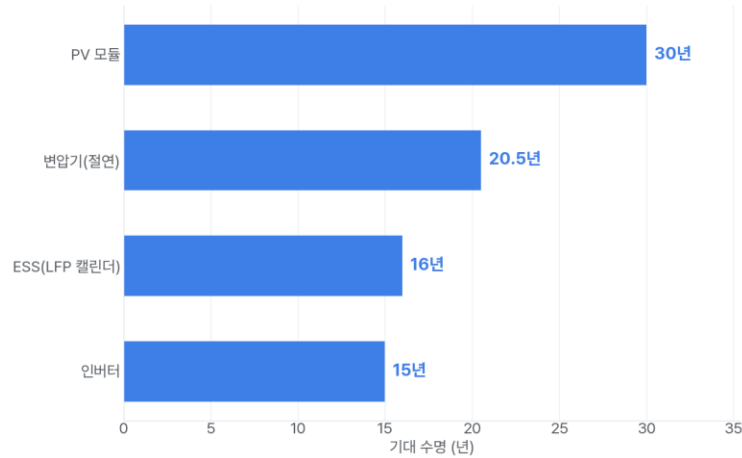
[그림 3] 설비별 기대수명(년): PV 모듈(NREL ATB 2024), 변압기 절연(IEEE C57.91), ESS LFP 셀린더(PNNL 2022), 인버터(BFH 2022)
