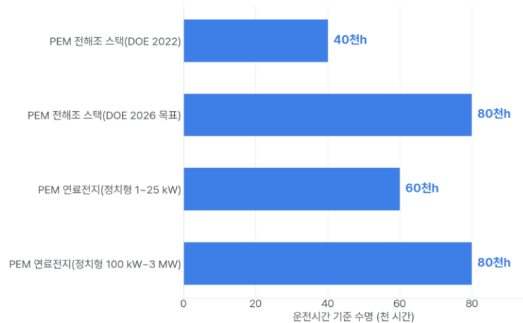
[그림 4] 스택 운전시간 기준 수명(천 시간): PEM 전해조(DOE 2022 현황·2026 목표), 정치형 PEM 연료전지(DOE 목표)
